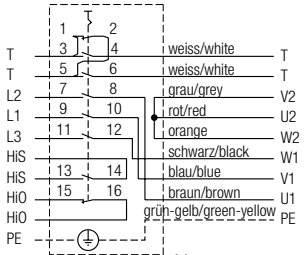
Netz Revisionschalter Mains Isolator Motor Y-Schaltung 400 V Y-Connection
