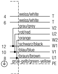
Motor \Delta -Schaltung 230 V \Delta -Connection
