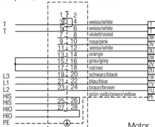
Netz/Mains hohe Drehzahl high speed Revisionsschalter Isolator
