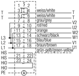
Netz Revisionsschalter Motor Δ Mains Isolator hohe Drehzahl/high speed
