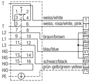
Netz Revisionsschalter Mains Isolator
